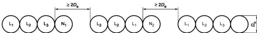
Рисунок Н.52.4 - Специальная конфигурация для девяти параллельных одножильных кабелей в горизонтальной плоскости
