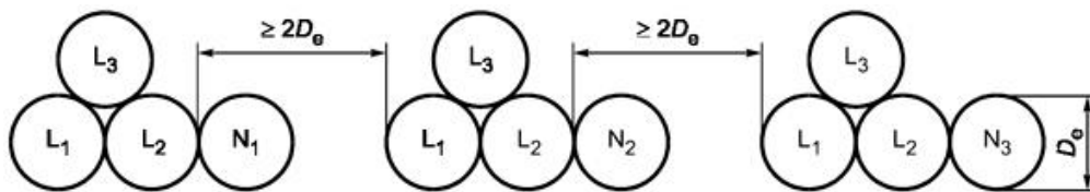
Рисунок Н.52.6 - Специальная конфигурация для девяти параллельных одножильных кабелей, уложенных треугольником
